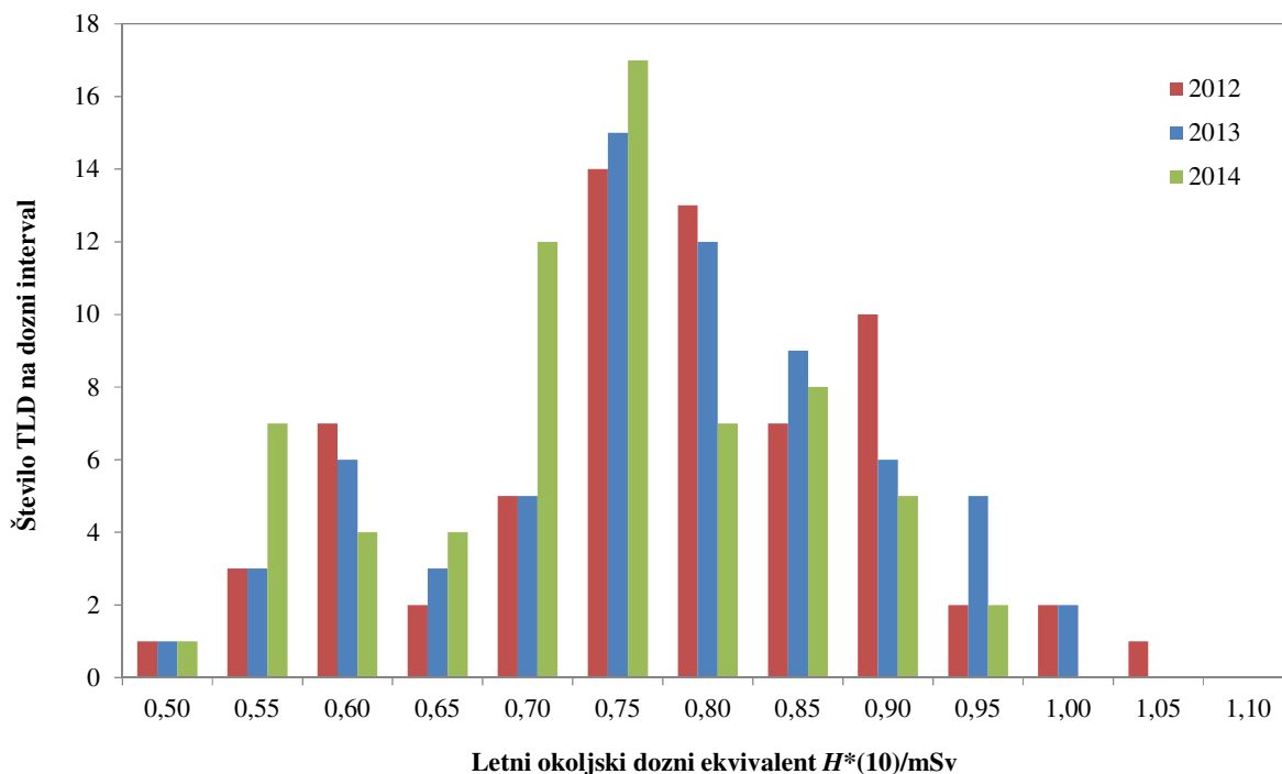
Slika 6.3: Porazdelitev letnega okoljskega doznega ekvivalenta, H^*(10) za vse dozimetre ( N = 67 ) na ograji NEK in v okolici NEK ter na referenčni lokaciji v Ljubljani po dozni intervalih 0,05 mSv v letih 2012, 2013 in 2014. Pri posameznem dozni intervalu je navedena srednja vrednost tega intervala (npr. za interval od 0,525 mSv do 0,575 mSv je to 0,55 mSv).
