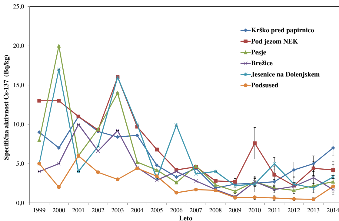
Slika 2.9: Primerjava specifičnih aktivnosti Cs-137 v talnem sedimentu reke Save. Merske negotovosti so v zadnjih letih od 0,3 Bq/kg do 2 Bq/kg.
