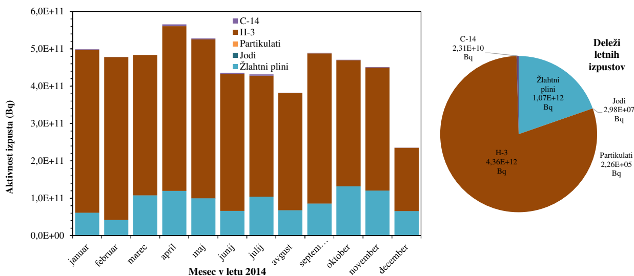
Slika 5.7: Mesečne inhalacijske in imerzijske doze za posameznika iz prebivalstva v naselju Spodnji Stari Grad (zgornji graf) in plinski izpusti NEK (spodnji graf), na podlagi katerih so te doze izračunane. Največji prispevek k inhalacijski dozi daje H-3 v obliki vodne pare, k imerzijski pa različni izotopi Xe in Ar-41 (Preglednica 5.2.).
