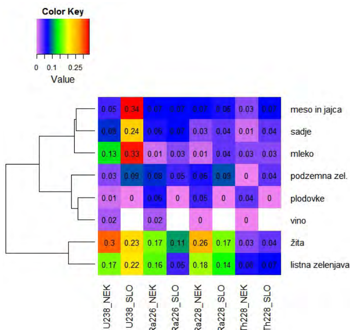
Slika 7.5: Izmerjene povprečne specifične aktivnosti U-238, Ra-226, Ra-228 in Th-228 (Bq/kg) v vzorčenih skupinah živil v letu 2014 v okolici NEK in drugod po Sloveniji
