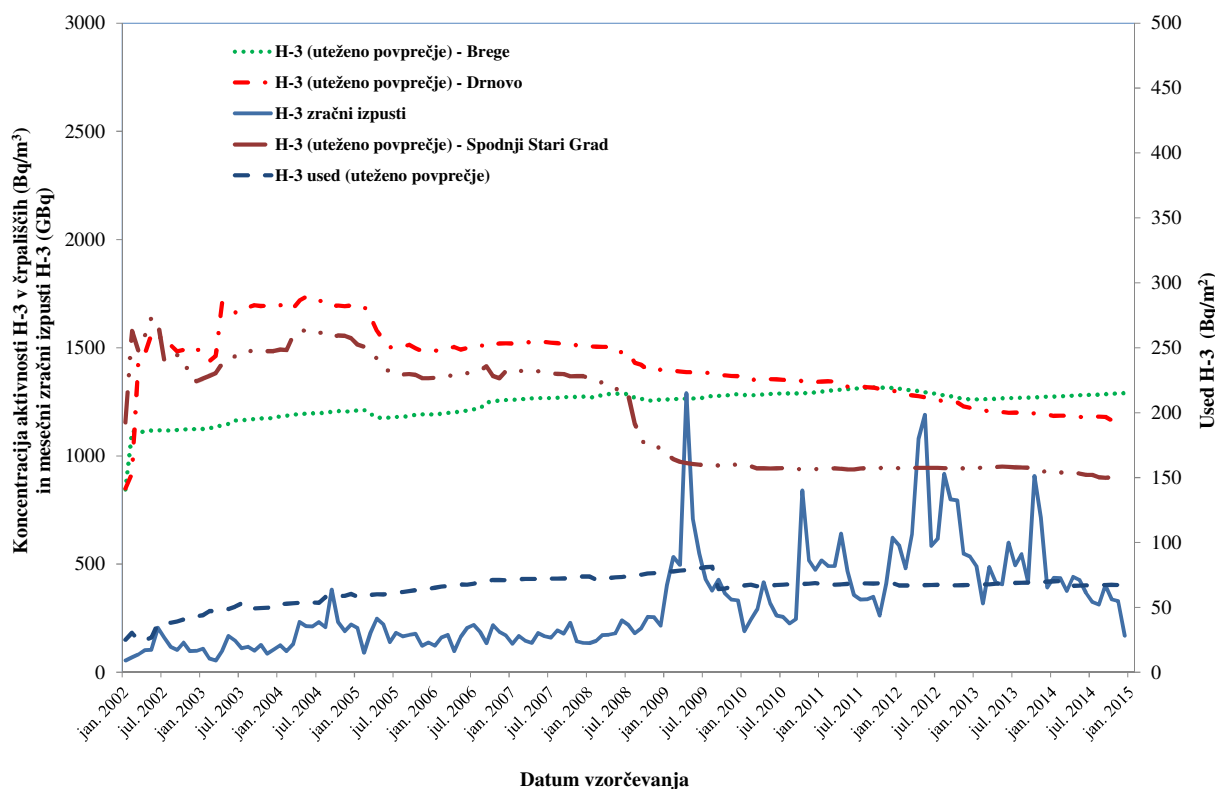
Slika 3.8: Primerjava med uteženim povprečjem koncentracije aktivnosti H-3 v pitni vodi (Brege in Drnovo), uteženim povprečnim usedom tritija v Bregah ( Bq/m^2 ) ter mesečnimi zračnimi izpusti od leta 2002 do 2014
