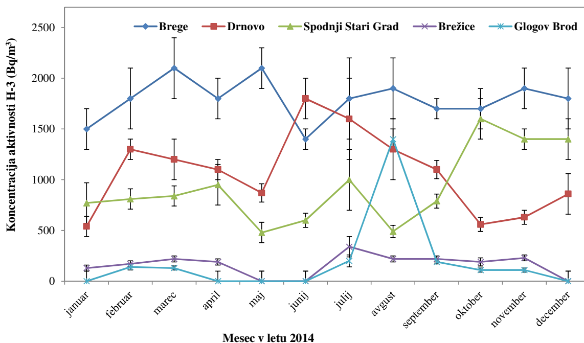
Slika 3.2: Mesečna koncentracija aktivnosti H-3 vzorcev pitne vode iz črpališč in vodovodov za leto 2014
