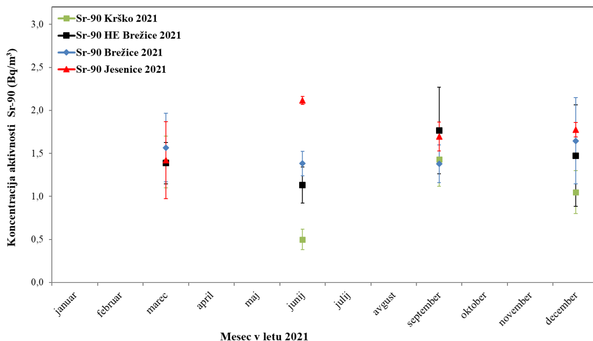
Slika 1.9: Primerjava četrtnih povprečnih koncentracij aktivnosti Sr-90 v vodi (v suhem ostanku po izparevanju vzorca) reke Save na lokacijah Krško, nad jezo HE Brežice, Brežice in Jesenice na Dolenjskem. Meritve na lokacijah nad jezo HE Brežice, Brežice in Jesenice na Dolenjskem so mesečne.
