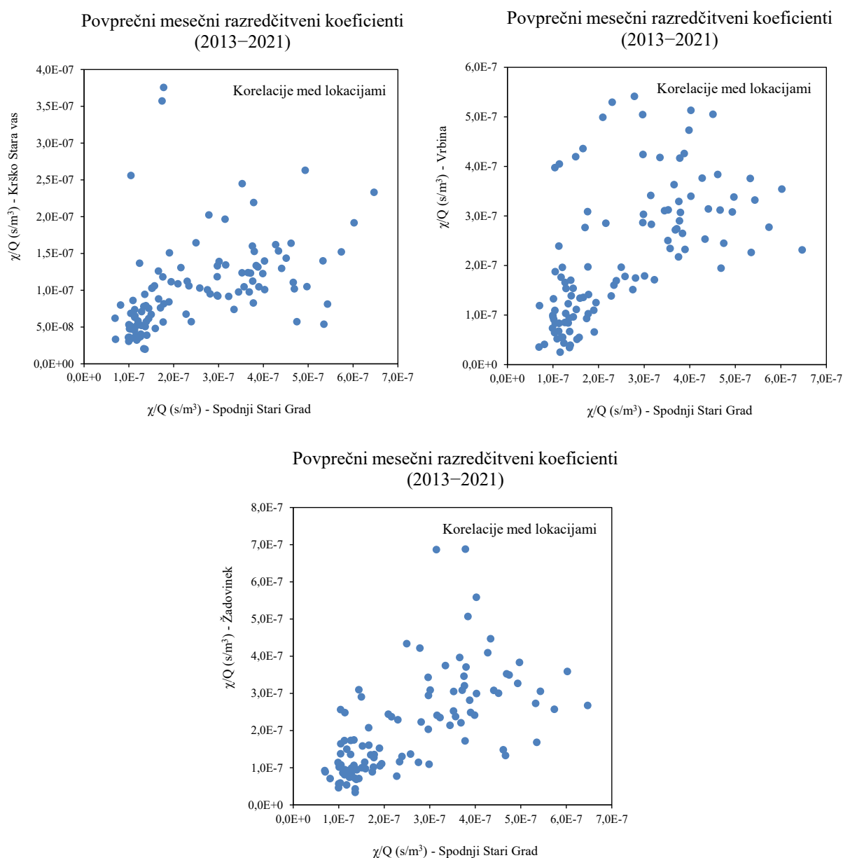
Slika 4.7: Korelacija povprečnih mesečnih razredčitvenih koeficientov ( \chi/Q ) z enoto s/m 3 , na referenčni lokaciji Spodnji Stari Grad in v bližnjih naseljih za leta 2013–2021.
