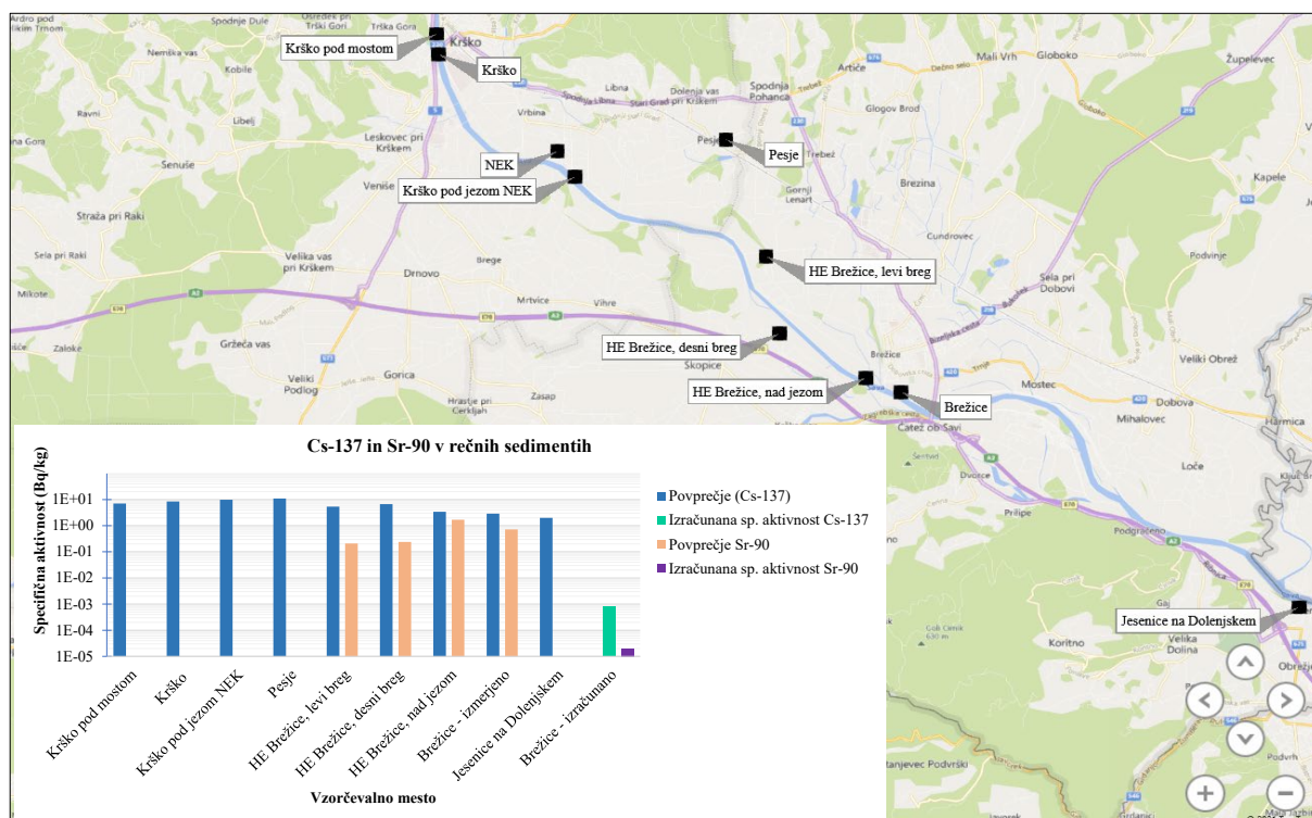
Slika I3: Specifične aktivnosti Cs-137 in Sr-90 v sedimentih v letu 2021. Povprečje Sr-90 v Krškem je bilo pod mejo detekcije. Skala je logaritemska.
