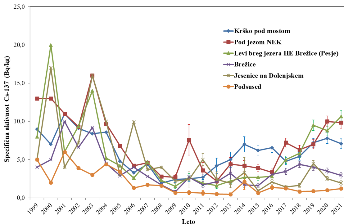
Slika 1.8: Primerjava specifičnih aktivnosti Cs-137 v talnem sedimentu reke Save na lokacijah vzdolžno in nizvodno od jezua NEK. Prikazane so povprečne specifične aktivnosti od 1999 do 2021.
