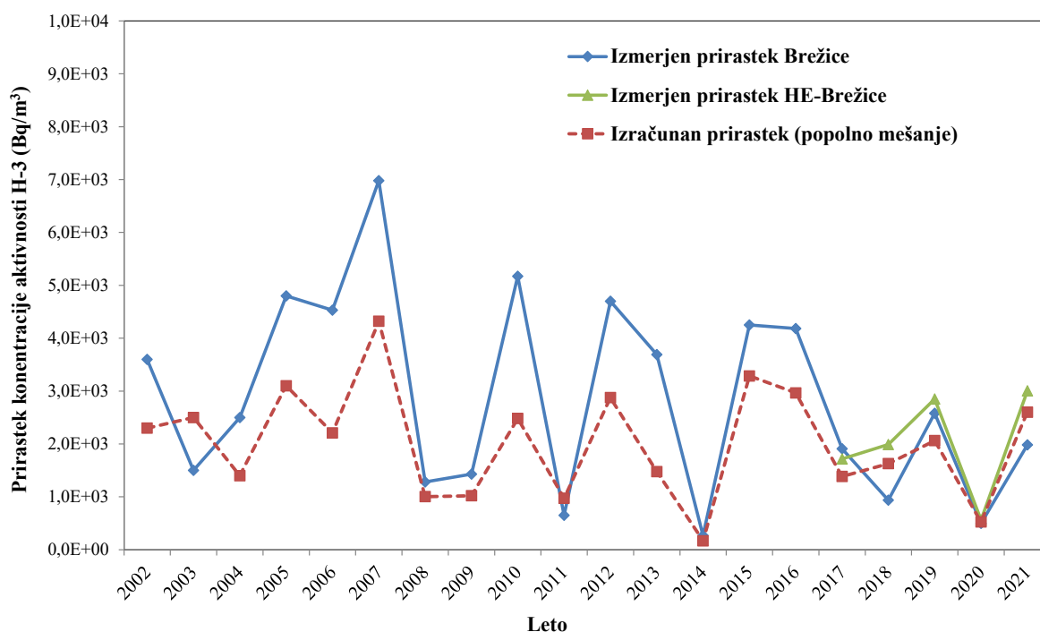
Slika 1.7: Primerjava med letnima povprečnima prirastkoma koncentracije aktivnosti H-3 v reki Savi na jezu HE Brežice ter za jezo v Brežicah in izračunano koncentracijo aktivnosti H-3, dobljeno iz letnih tekočinskih izpustov in pretoka Save ob predpostavki popolnega mešanja
