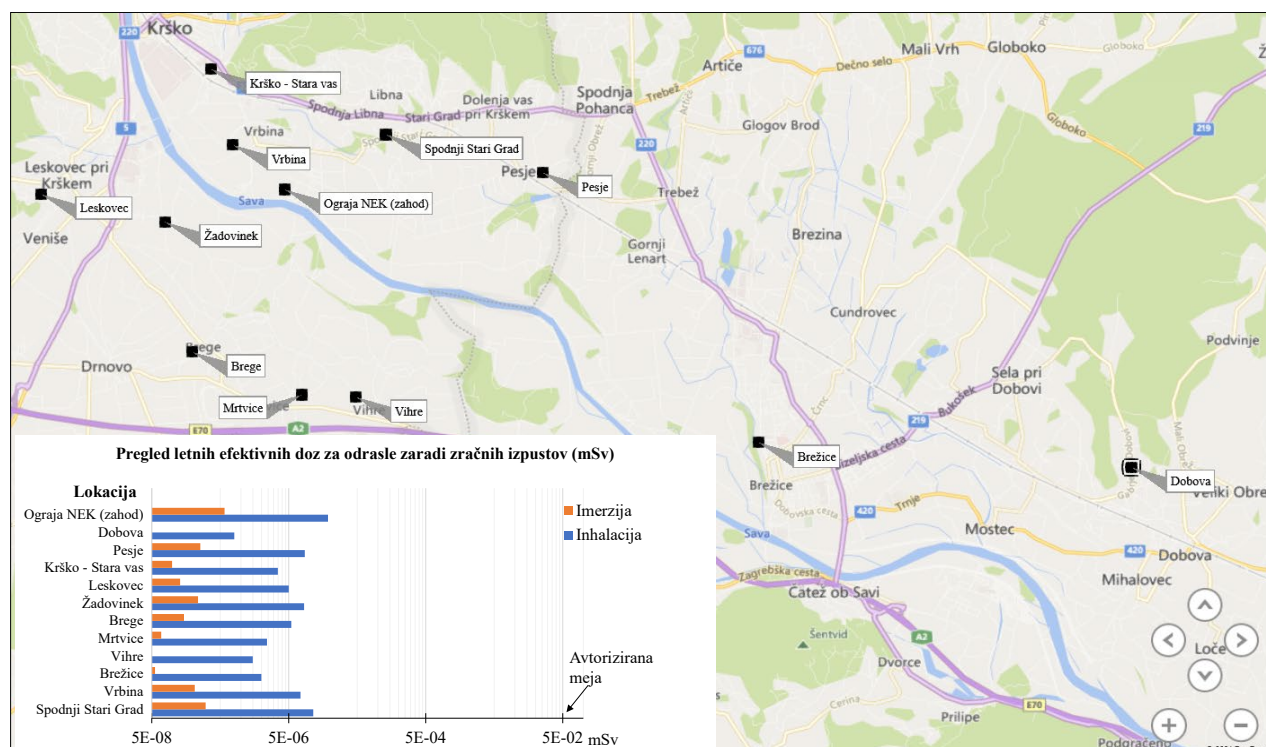
Slika P1: Pregled ocenjenih letnih efektivnih doz za umetne radionuklide za zračne izpuste v okolici NEK v letu 2021. Ocena učinka na prebivalstvo je bila narejena na podlagi meritev zračnih izpustov (emisij) in z uporabo razredčitvenih faktorjev Lagrangeevega modela. Skala na legendi je logaritemska.
