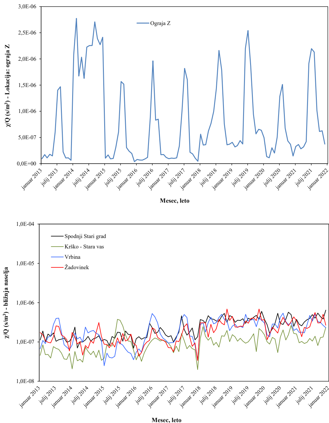
Slika 4.6: Povprečni mesečni razredčitveni koeficienti ( \chi/Q ) z enoto s/m^3 , izračunani po Lagrangeevem modelu za izpust z višine 60 m za okolico NEK za leta 2013–2021.
